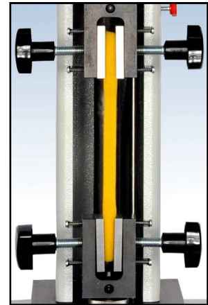
Schraubklemmen
