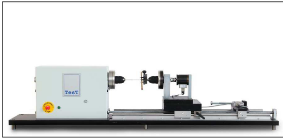
Kombinierte Prüfmaschine mit gleichzeitiger Axial- und Torsionsbelastung
