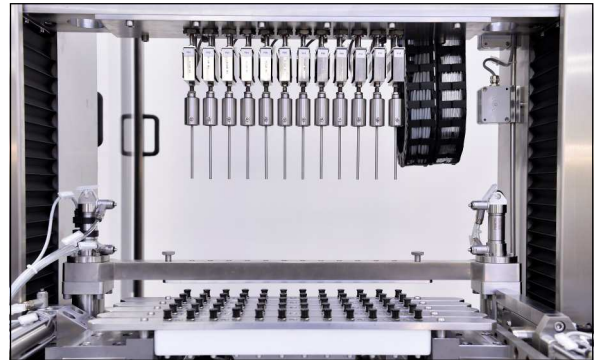
Prüfung von Injektions-Ampullen (Medizintechnik)
