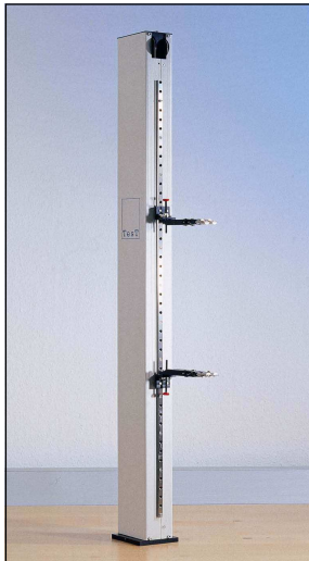
Langweg- Dehnungsaufnehmer
